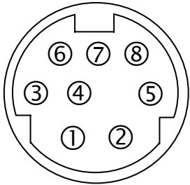
8PIN male Mini Din (up view of cable)
